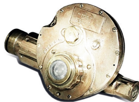
Прицел 76-мм корабельного орудия Mk II 3°50 Mark 21 транспорта «Томас Дональдсон»
